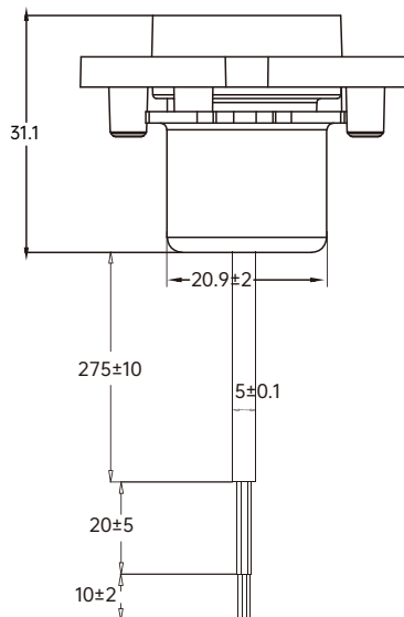
Receptacle
